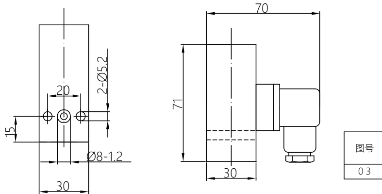
505-18D O型密封圈尺寸: \phi 5 \times 15 订货目录编号: 0664098
